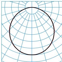
Olisq QWD2 DW 20-840 ETBLE +DMR IP54 + Olisq QWD2 ZDR 1/1 03 TX461452
