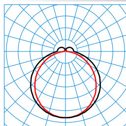
Olisq LWD3 DW 75-830 ET2 IK TX564729
