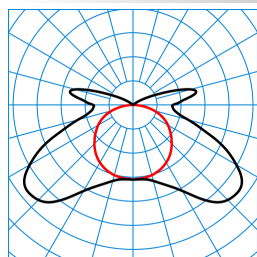
AragF 15 PXW 64-840 ETDD +HFSB LV PC TX782512
