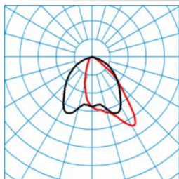
Jovie 70-AM3L-18-180-740-CLO-B
