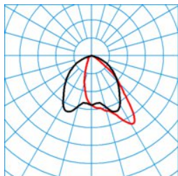
Jovie 70-AM3L-18-180-740-CLO-E
