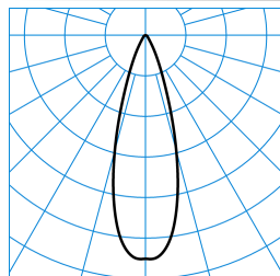
LnStar 40-RE2L/3200-740 4G1S ET TX779681
