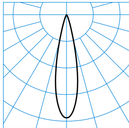
7651 Lentyp L-SP 40-EW M48 ETBLE 05 (225) TX782453
