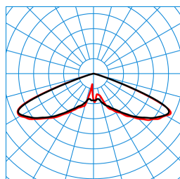
Publisca P1W-RB6L-LRA/2600-740 3G1S ET (CLO initial value) TX300517
