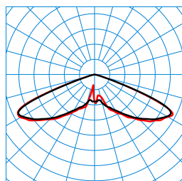
Publisca P1W-RB6L-LRA/2600-740 3G1S ET (CLO end value) TX300971
