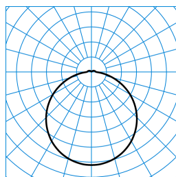
Olisq RWD2 DW 40-840 ET2 IP54 + Olisq RWD2 C 01 TX425844
