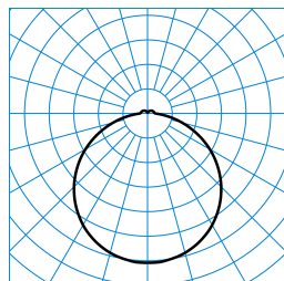
Olisq RWD2 DW 40-840 ET2 IP54 + Olisq RWD2 ZDR 1/2 05 TX428732
