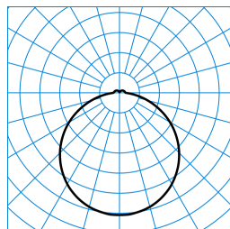
Olisq RWD2 DW 40-840 ET2 IP54 + Olisq RWD2 ZDR 1/2 03 TX427818
