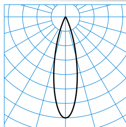
7651 Lentyp L-MF 40-EC M39 ET 01 (150) TX782121
