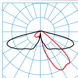
8841LS-UE 260-AB2L/1000-730 2G2 ET (CLOANFANGSWERT) TX778494
