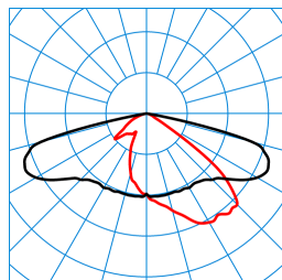
US 9711-AB7L-LR/220/260/320-740 4G1 (3200 lm) TX055677
