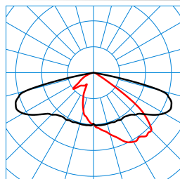
US 9711-AB7L-LR/220/260/320-740 4G1 (2200 lm) TX055663
