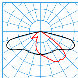
US 9711-AB7L-LR/220/260/320-740 4G1 (2600 lm) TX055664
