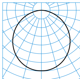
Olisq RWD2 DW 20-840 ETBLE +CAS-S + Olisq RWD2 ZDR 1/1 01 TX565742
