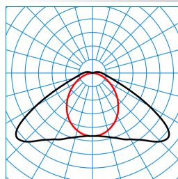
Nextrema G3 XB 6000-840 ET +LV TX770680
