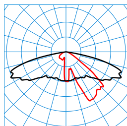
Publisca P1W-AB2L-LRA/1200-740 2G1S ET (CLO end value) TX300680
