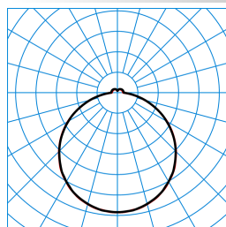
Olisq QWD3 DW 30-830 ET EB3 IP54 IK TX778180
