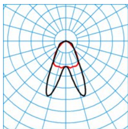
ELINE LDAN55-140 ML 840 L225 2 50 ■ C0 - C180
