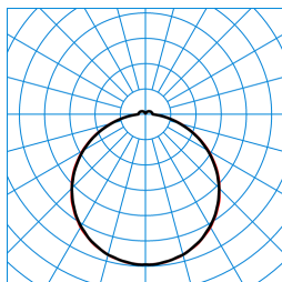
Olisq QWD3 DW 45-830 ETBLE +DMR IP54 + Olisq QWD3 ZDR 1/2 03 TX461281
