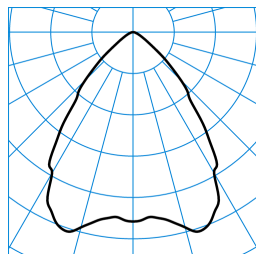
InperiaLP C05 BR22 1800-840 01 + RD-PC TX041247 ■ C0 - C180
