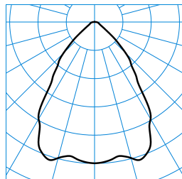
InperiaLP C05 BR22 1800-840 01 + ZN-PC TX041249 ■ C0 - C180
