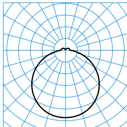
Olisq RWD1 DW 10-840 ETDD IP54 + Olisq RWD1 ZDR 1/2 03 TX425807
