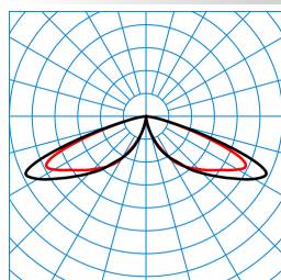
LTX PT-RB6L-LR/1800-730 2G1 ET TX779703
