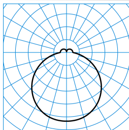
Olisq RWD1 DW 20-830 ET IP54 PC TX376297
