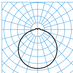
Olisq RWD1 DW 20-830 ET IP54 PC + Olisq RWD1 ZDR 1/2 01 TX425677
