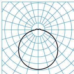
Olisq RWD1 DW 20-830 ET IP54 PC + Olisq RWD1 C 01 TX425613
