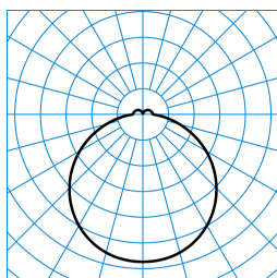
Olisq RWD1 DW 20-830 ET IP54 PC + Olisq RWD1 ZDR 1/2 05 TX428861
