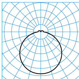
Olisq RWD1 DW 20-830 ET IP54 PC + Olisq RWD1 ZDR 1/2 03 TX429095
