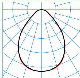
ArmoFit G2 M59 PW19 53-940 ET + ArmoFit G2 Sky M59-TS ZER TX426834
