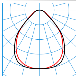
ArmoFit G2 M59 PW19 53-940 ET TX376400
