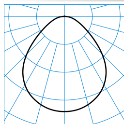
Onplana D09 CDP19 2000-830 ET 26 TX771785
