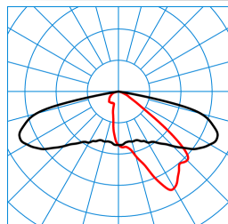
Cuvia 40-AB2L/2600-740 4G1S ET TX775984
