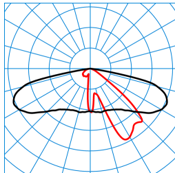
Publisca P1-AB2L/1800-740 2G1S ETDD (CLO initial value) TX300588
