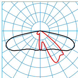
Publisca P1-AB2L/1800-740 2G1S ETDD (CLO end value) TX300797
