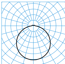
Olisq RWD2 DW 20-830 ETBLE +CAS IP54 + Olisq RWD2 ZDR 1/2 05 TX565845
