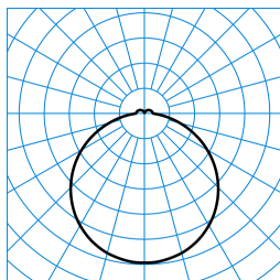
Olisq RWD3 DW 50-840 ET IP54 + Olisq RWD3 ZDR 1/2 03 TX426729
