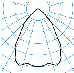
InperlaLP C05 BR22 1800-840 03 + ZN-PC TX041555 ■ C0 - C180
