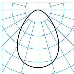
InperlaLP C05 BR22 1800-840 03 + DA-M 01 TX041551 ■ C0 - C180
