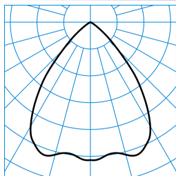
InperlaLP C05 BR22 1800-840 ETDD 03 TX771524 ■ C0 - C180
