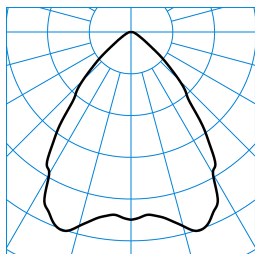
InperlaLP C05 BR22 1800-840 03 + RG-PC TX041554 ■ C0 - C180
