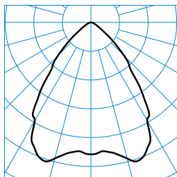
InperlaLP C05 BR22 1800-840 03 + RD-PC TX041553 ■ C0 - C180
