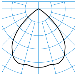
InperlaL G2 C07 BR22 1800-840 EB3 01 + RG-PC ■ C0 - C180 TX052897
