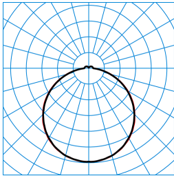
Olisq QWD2 DW 14-40/4/ML-840 IP54 IK ET + Olisq QWD2 ZDR 1/2 01 (stage 1) TX461116
