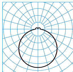
Olisq QWD2 DW 14-40/4/ML-840 IP54 IK ET (stage 2) TX777311
