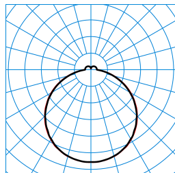
Olisq QWD2 DW 14-40/4/ML-840 IP54 IK ET (stage 1) TX777309
