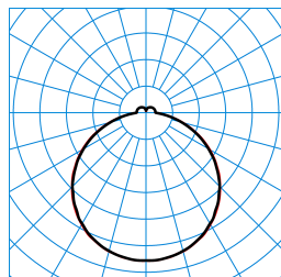
Olisq QWD2 DW 14-40/4/ML-840 IP54 IK ET (stage 3) TX777313
