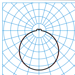
Olisq QWD2 DW 14-40/4/ML-840 IP54 IK ET (stage 0) TX777306
