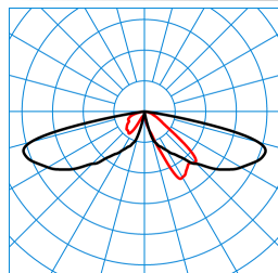
LTX P-AB2L-LRA/1800-740 2G1 ETDD TX779368
