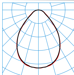
ArimoFit M48 PW19 53-840 ET TX429026
