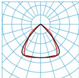
ELINE HE LW2260-160 ML 865 L225 0 20 ■ C0 - C180
