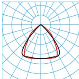
ELINE HE LW2260-160 ML 865 L225 2 20 ■ C0 - C180
