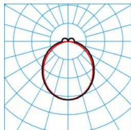
ELINE DSL50-130 ML 830 L225 4 50
