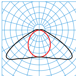
Nextrema G3 XB 40-840 ET +LV TWP PC TX769940
