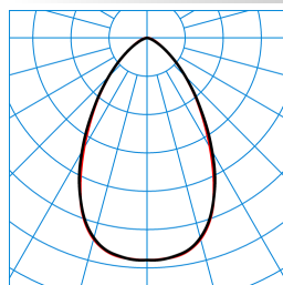
Mirona Fit 4L BS TB 260-840 ET TX771144
