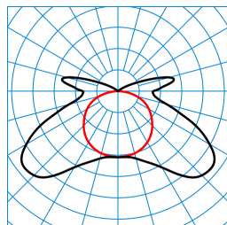
AragF 12 PXW 20-65/16ML-840 ET (stage 15) TX770021
