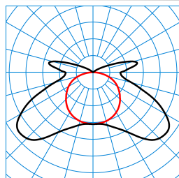
AragF 12 PXW 20-65/16ML-840 ET (stage 0) TX769759
