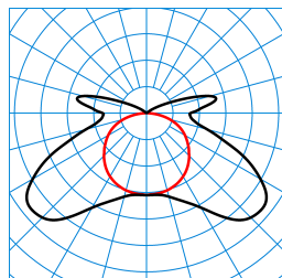
AragF 12 PXW 20-65/16ML-840 ET (stage 1) TX769756
