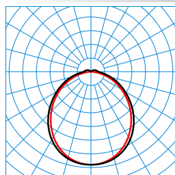
4401 G2 C15 DW IP 40-840 ETDD TX773652
