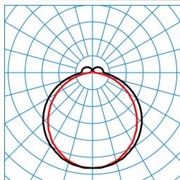
Olisq LWD2 DW 20-60/4/ML-830 ET IP54 IK (stage 1) TX564640
