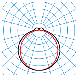
Olisq LWD2 DW 20-60/4/ML-830 ET IP54 IK (stage 2) TX564641
