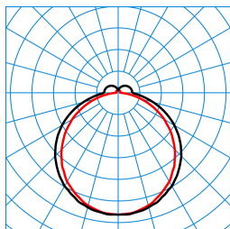
Olisq LWD2 DW 20-60/4/ML-830 ET IP54 IK (stage 3) TX564642
