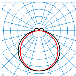
Olisq LWD2 DW 20-60/4/ML-830 ET IP54 IK (stage 4) TX564643
