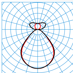
Opendo H2-L PW19 64-840 ETDD +EB3 03 TX277423
