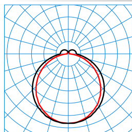
Olisq LWD1 DW 20-840 ET IP54 TX376044
