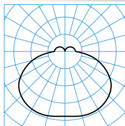
PolaronIQ WD1-2D LED3000-830 ET TX773770
