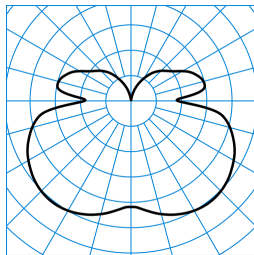
PolaroniQ H2D LED2000-840 ET 1,0m TX773845
