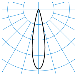
7651 LentyP L-SP 30-EW M48 ET 05 (225) TX782447
