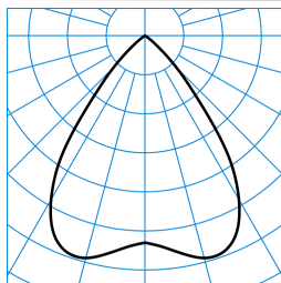
InperiaL G2 C07 BR19 1800-840 ET 03 ■ C0 - C180 TX768209
