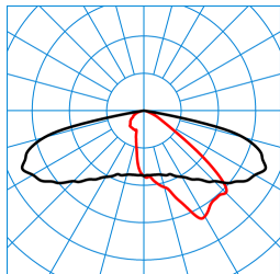
LIQ 50N-AB2L-LR/3200-722 4G1 ET (CLO end value) TX777713
