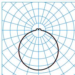
Olisq QWD2 DW 35-830 ETBLE +DMR IK TX777209
