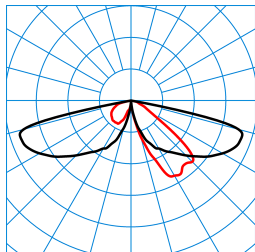
CS 19 100-AB2L-LR/5100-730 4G1S ET (CLO initial value) TX300035
