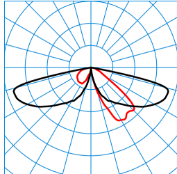
CS 19 100-AB2L-LR/5100-730 4G1S ET (CLO end value) TX300034
