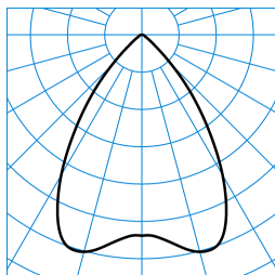
InperiaL G2 C07 HR19 1800-840 03 + RD-PC TX053022 ■ C0 - C180
