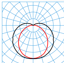
Kratex HE 1200 110-840 ET PC TX263562
